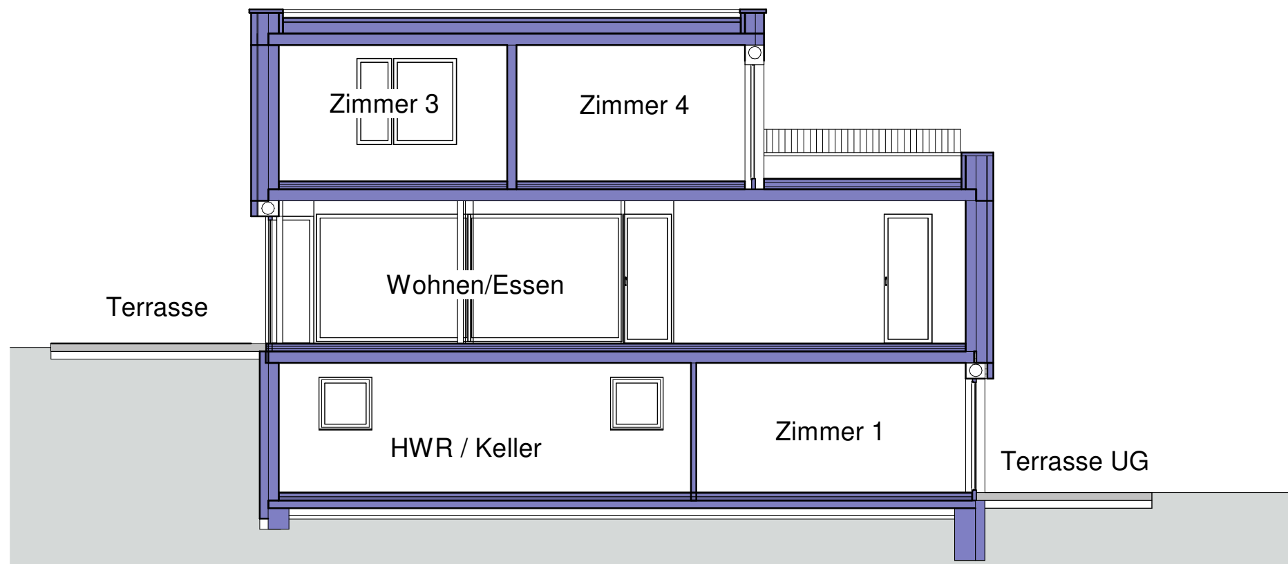
Schnitt S2
